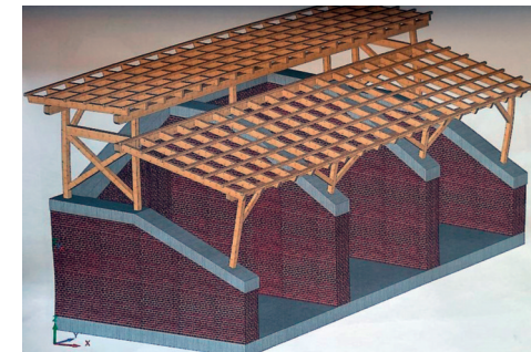
Weiterbau Gipsbrennofen vor der Niedtalhalle: Dachkonstruktion auf das vorhandene Mauerwerk
